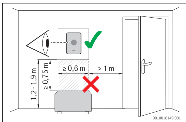
Afb. 3 Afstand voor de installatieplaats van de thermostaat
