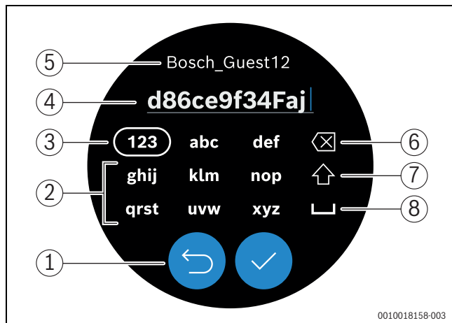
Afb. 12 Scherm WLAN-netwerkwachtwoord
