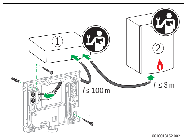
Afb. 6 Aansluiten van de adapter van de EasyControl
