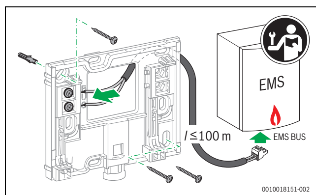
Afb. 5 Aansluiten van de muurplaat
