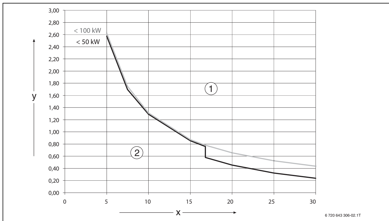
Afb. 1 Eisen aan het vul- en bijvulwater voor cv-toestellen met warmtewisselaar van aluminium materialen < 100 \text{ kW}
