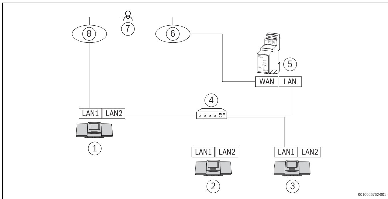
Afb. 44 Voorbeeld van een regelaarkoppeling met afstandsbediening en gebouwautomatiseringstechniek
