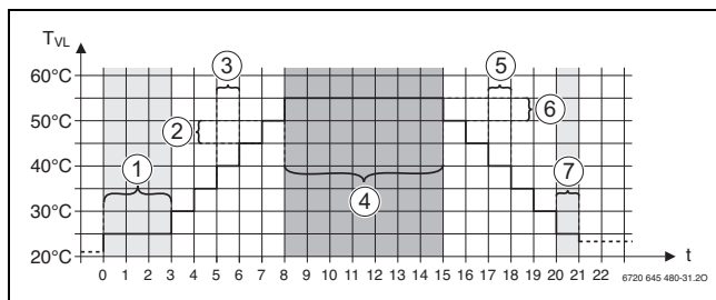
Afb. 41 drogen afwerkvloer
