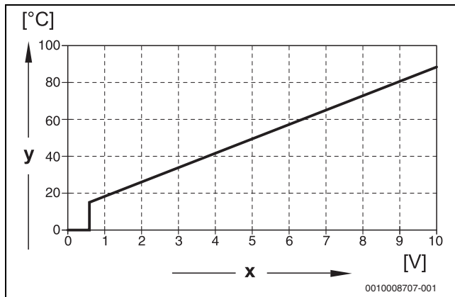
Afb. 25 0...10-V-ingang Temperatuur
