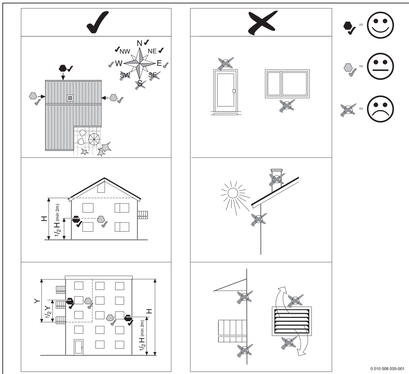
Afb. 7 Buitentemperatuursensor monteren
