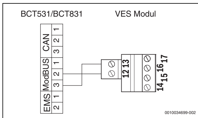
Afb. 34 Aansluiting van de regelaar aan de VES-module
