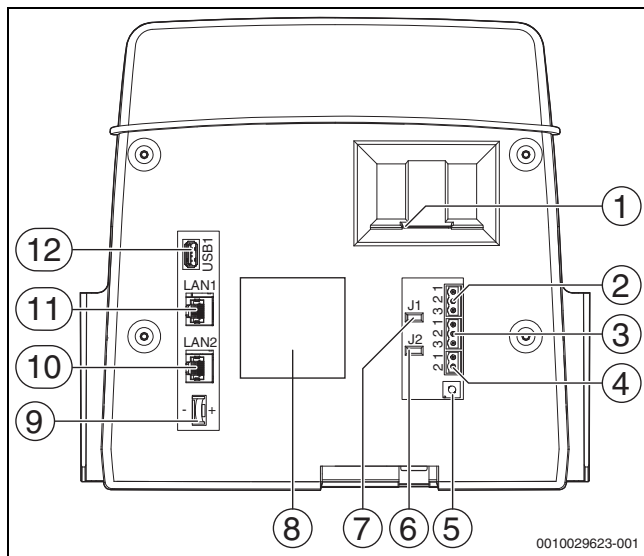
Afb. 4 Aansluitingen bedieningsunit
