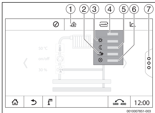
Afb. 39 Bedrijfsmodi
