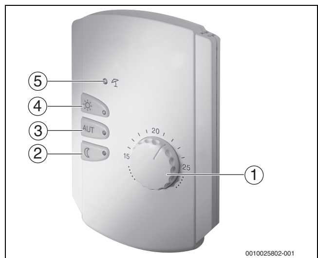
Afb. 36 Afstandsbediening
