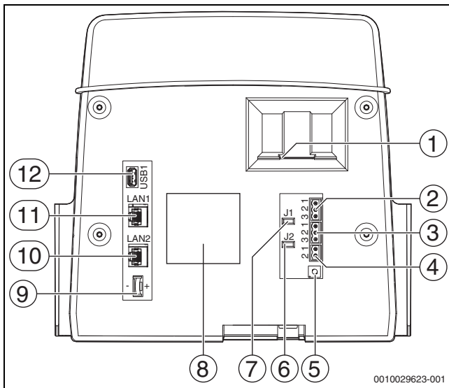
Afb. 22 Achterzijde bedieningsunit
