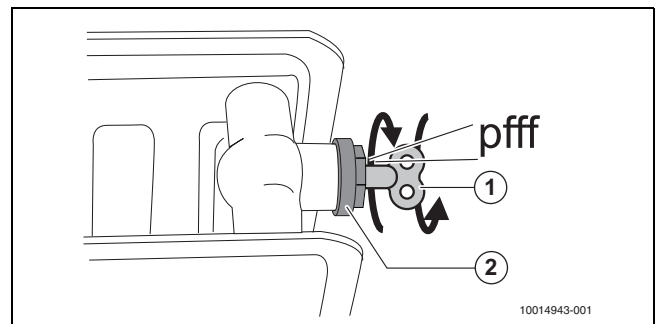
Afb. 9 Ontluchten radiator
