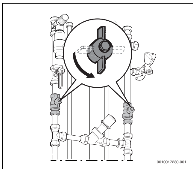
Afb. 4 Serviceafsluiters
