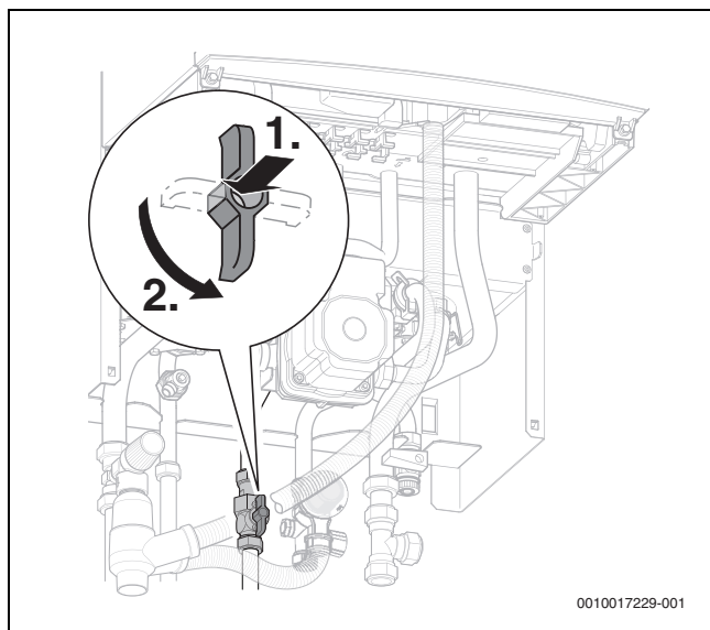
Afb. 3 Gaskraan
