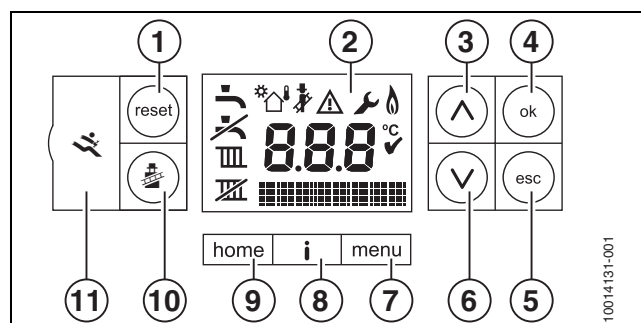
Afb. 5 Bedieningspaneel
