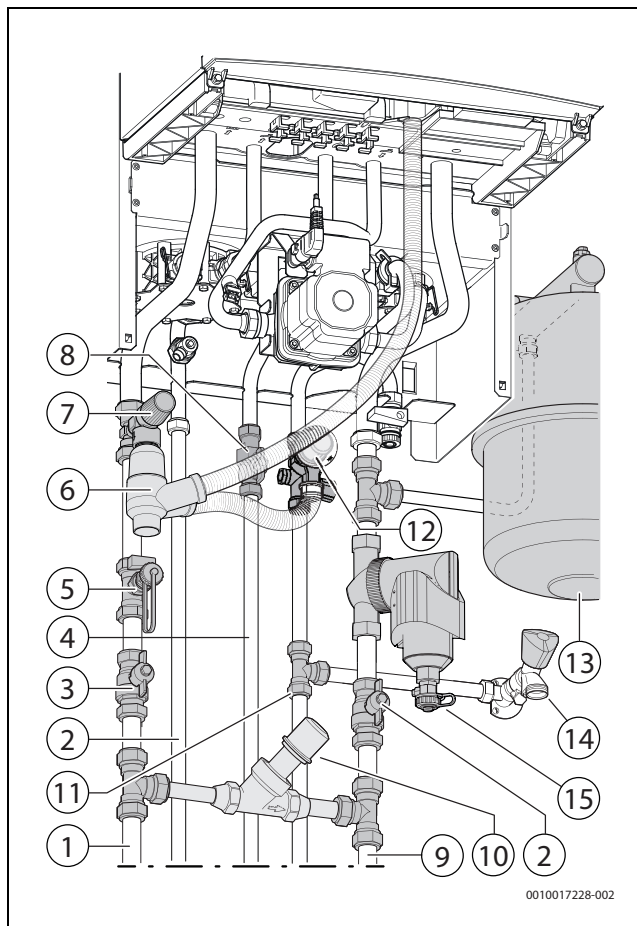
Afb. 2 Overzicht aansluitingen
