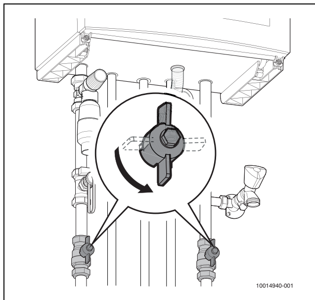
Afb. 4 Serviceafsluiters
