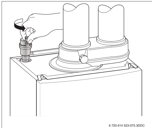
Afb. 7 Automatische ontlufter
