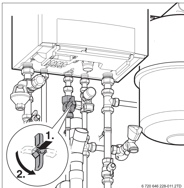
Afb. 3 Gaskraan
