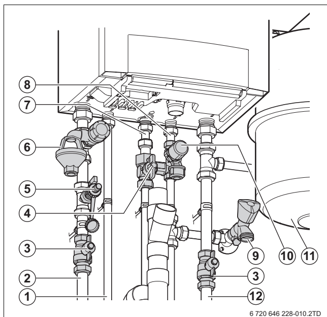
Afb. 2 Overzicht aansluitingen
