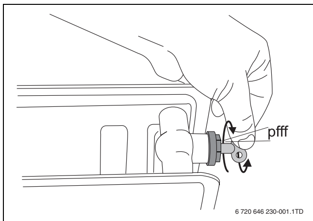
Afb. 8 Ontluchten radiator
