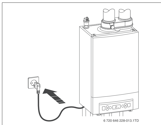
Afb. 5 Netstekker insteken
