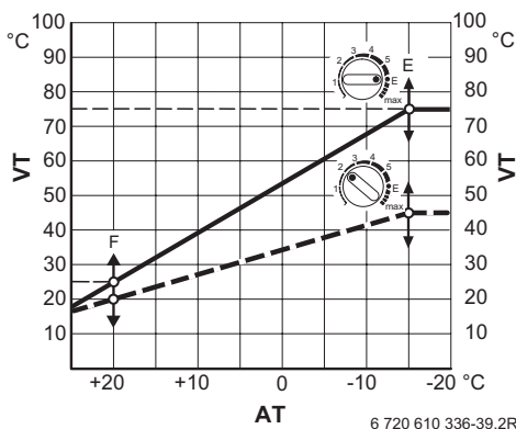
Afb. 14 Verwarmingscurve
